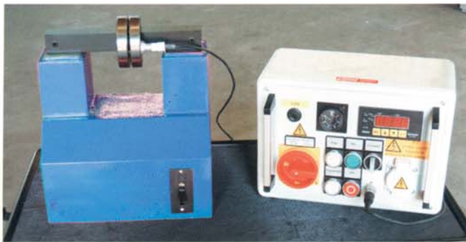
Induktives Aufheizen von Lagern aller Art Induction heating of all sorts of bearings
